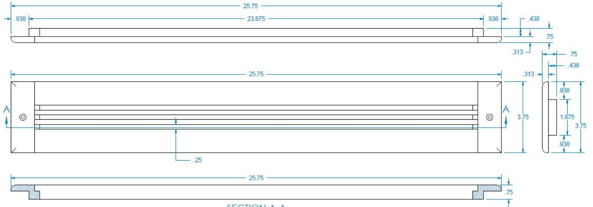
SECTION A-A
